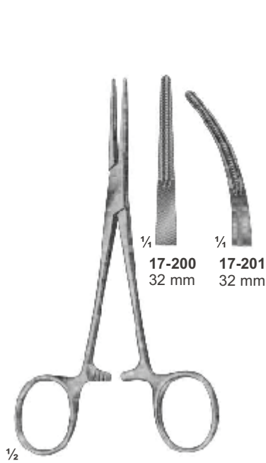
17-200 - 201 DE-BAKEY-KELLY 140 mm
