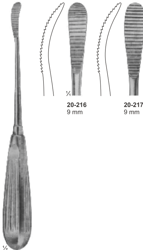
1/2 20-216 AUFRICHT up stroke 20-217 down stroke 220 mm
