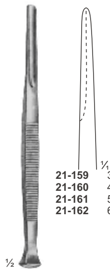
PARTSCH 21-159 - 162 Gouges 140 mm
